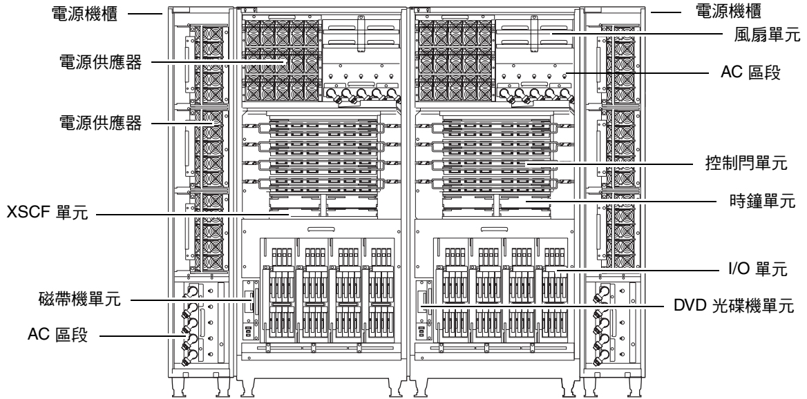
圖 1-8 M9000 (含擴充機櫃) 和電源機櫃正面圖
