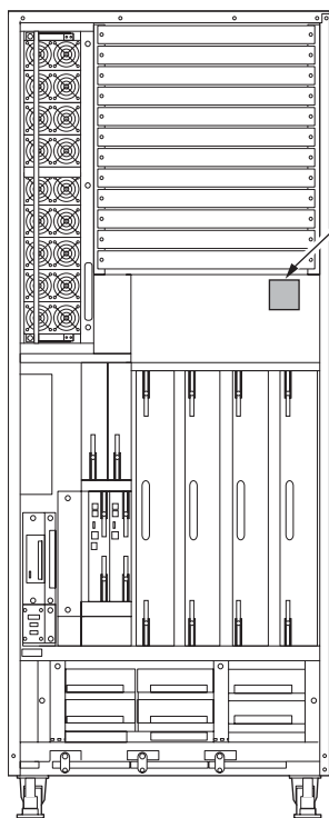
SPARC Enterprise M8000 伺服器 (正面視圖)
