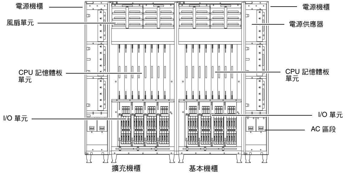
圖 1-9 M9000 (含擴充機櫃) 和電源機櫃背面圖
