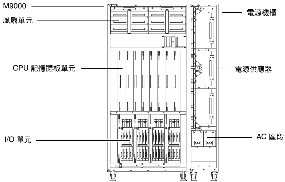
圖 1-7 M9000 (僅基本機櫃) 和電源機櫃背面圖
