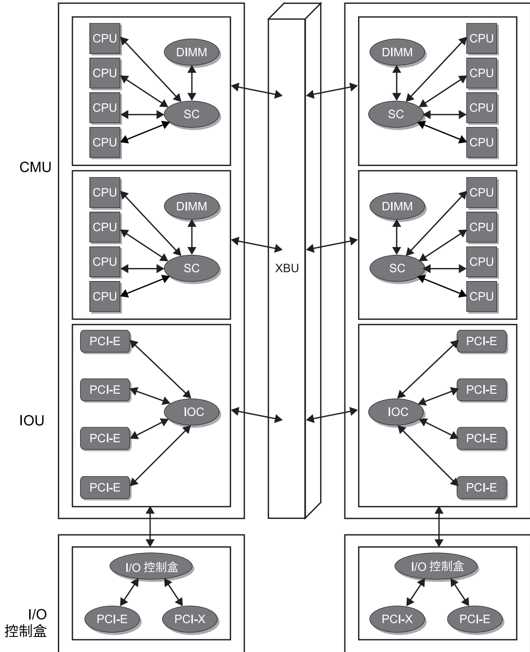
圖 2-1 主要元件連線
