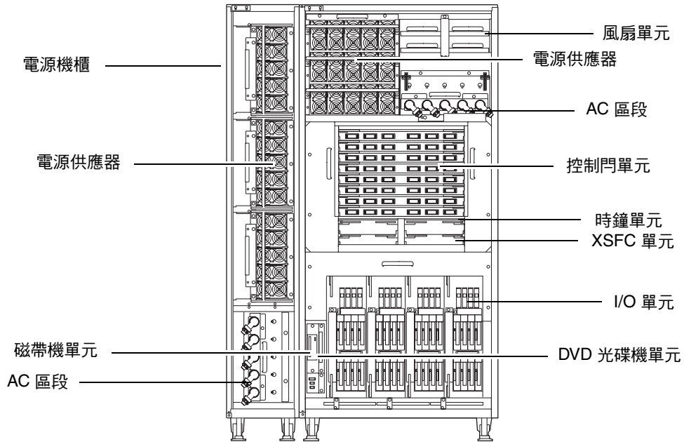
圖 1-6 M9000 (僅基本機櫃) 和電源機櫃正面圖
