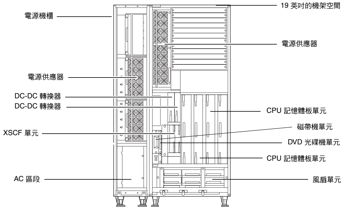
圖 1-4 M8000 和電源機櫃正面圖
