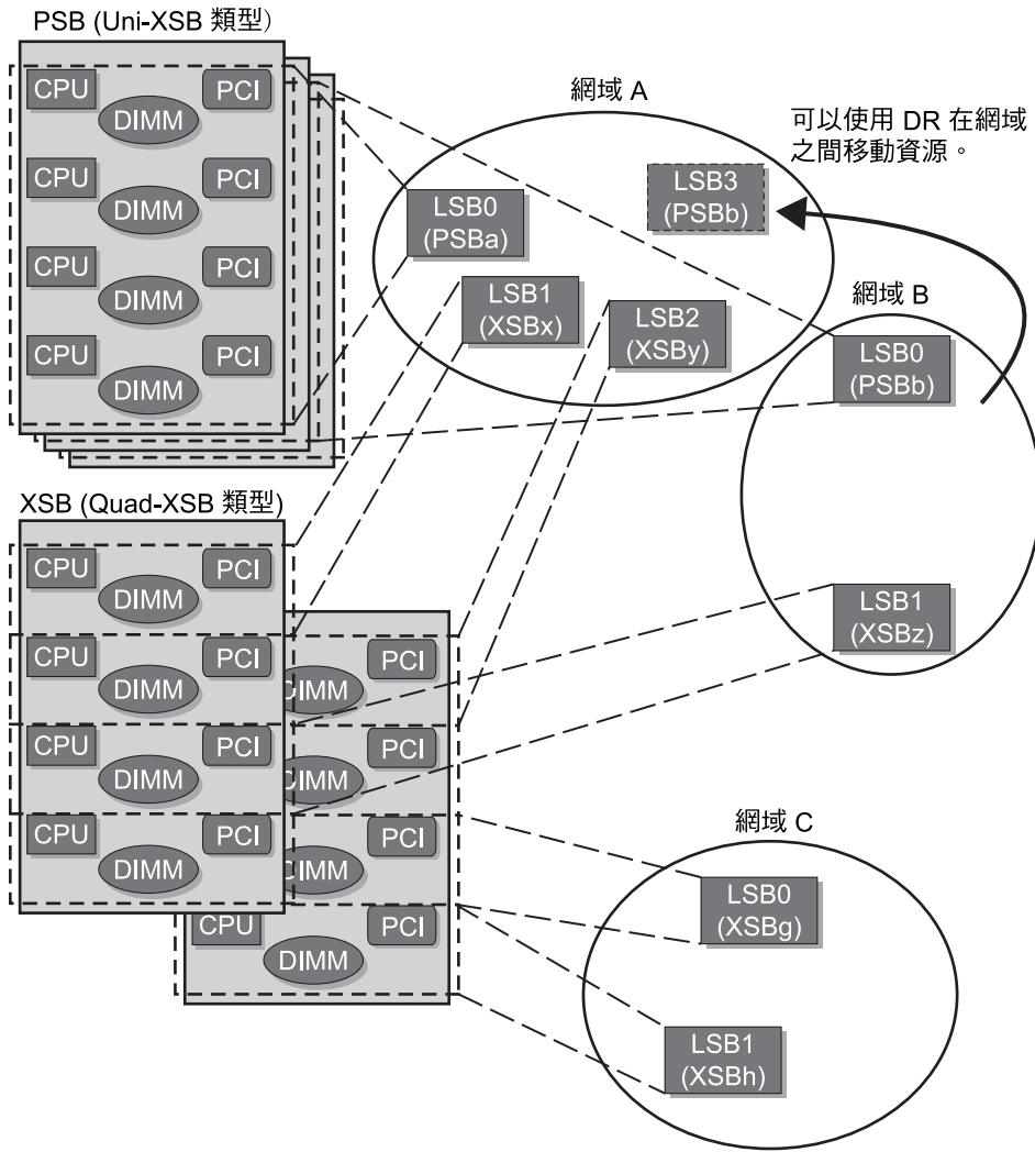
圖 2-3 網域配置
