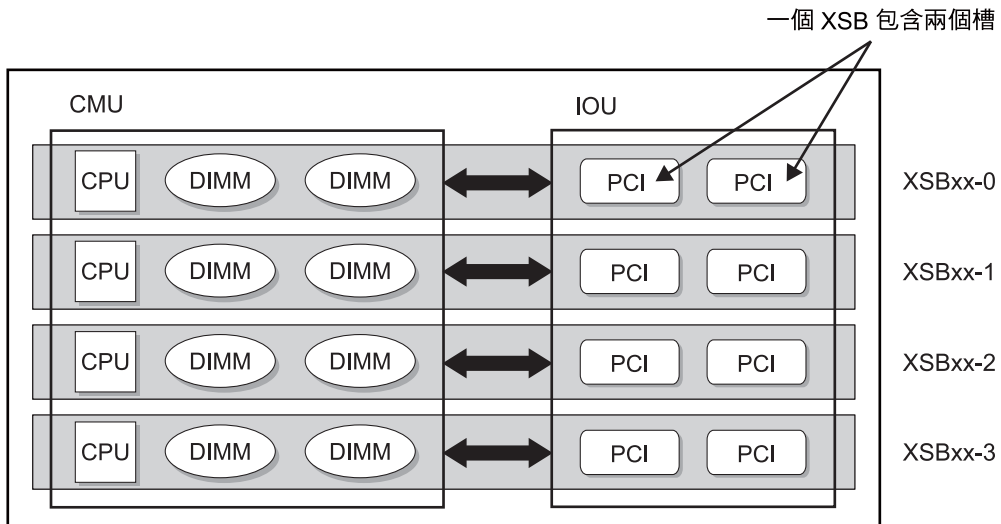
圖 2-2 分割區分割類型
