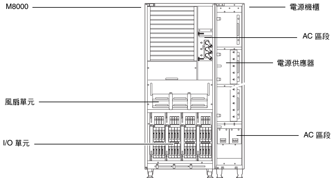
圖 1-5 M8000 和電源機櫃背面圖
